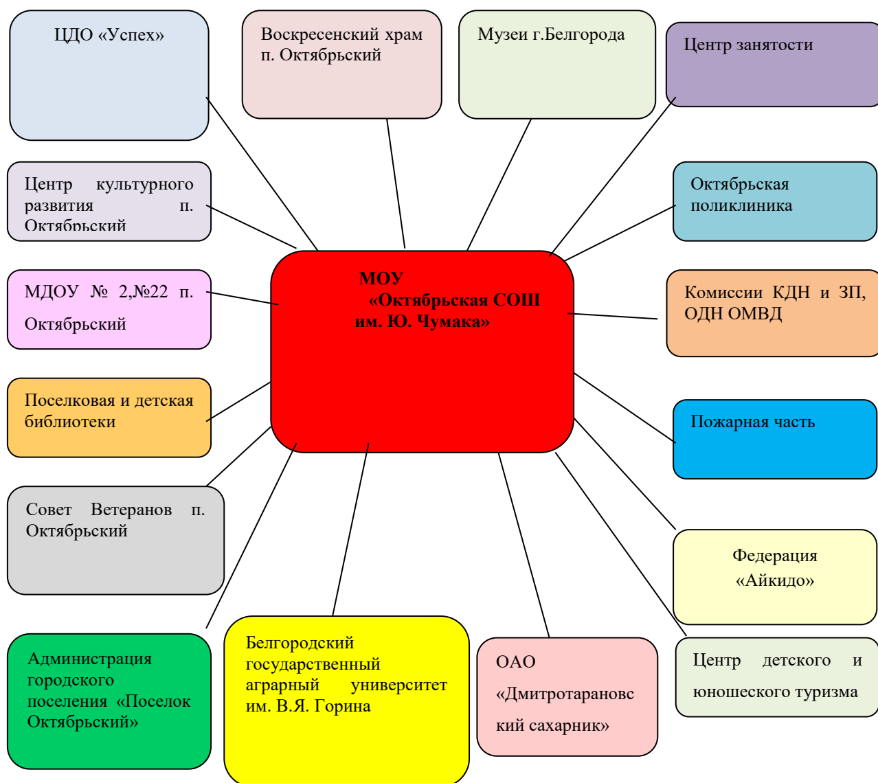
Схема 1.
